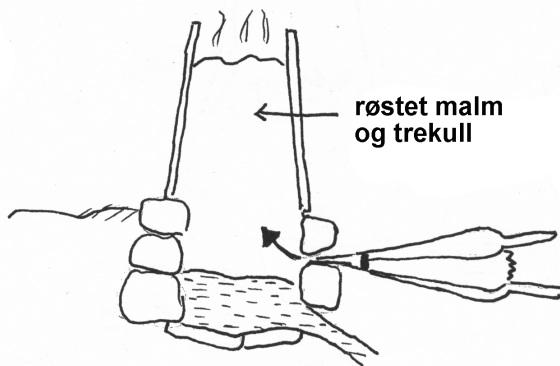
Sjaktovn med slaggavtapping Fra omkr. 600 til 1300-tallet
