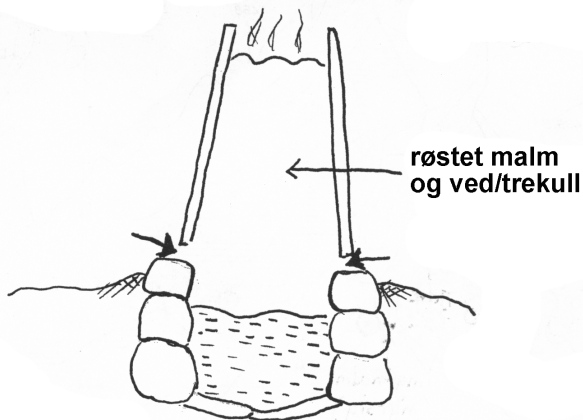
Sjaktovn med slaggopsamling i bunnen. Fra omkring Kr.f. til 500-tallet
