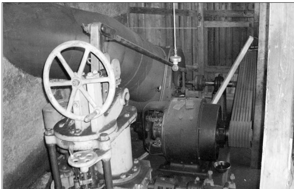
Fra turbinrommet. Rattet ble brukt til å regulere vanntilstrømmingen.
